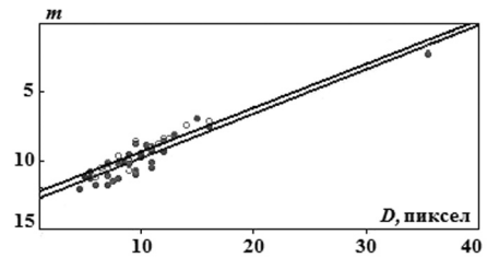
Рис. 6. Предельный блеск звезд для 200-мм объектива
