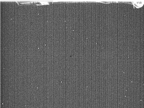
Рис. 3. Композитное изображение области Кассиопея-Персей-Андромеда на 1/3" матрице камеры КРС-650ВН с широкоугольным объективом (крестик-центр кадра, выделен «горячий пиксел»)
