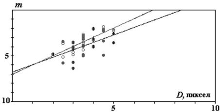
Рис. 4. Аппроксимация зависимости диаметр изображений ( D ) – блеск ( m ) прямыми
